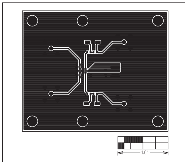
图3. MAX9583评估板PCB布局——元件层
