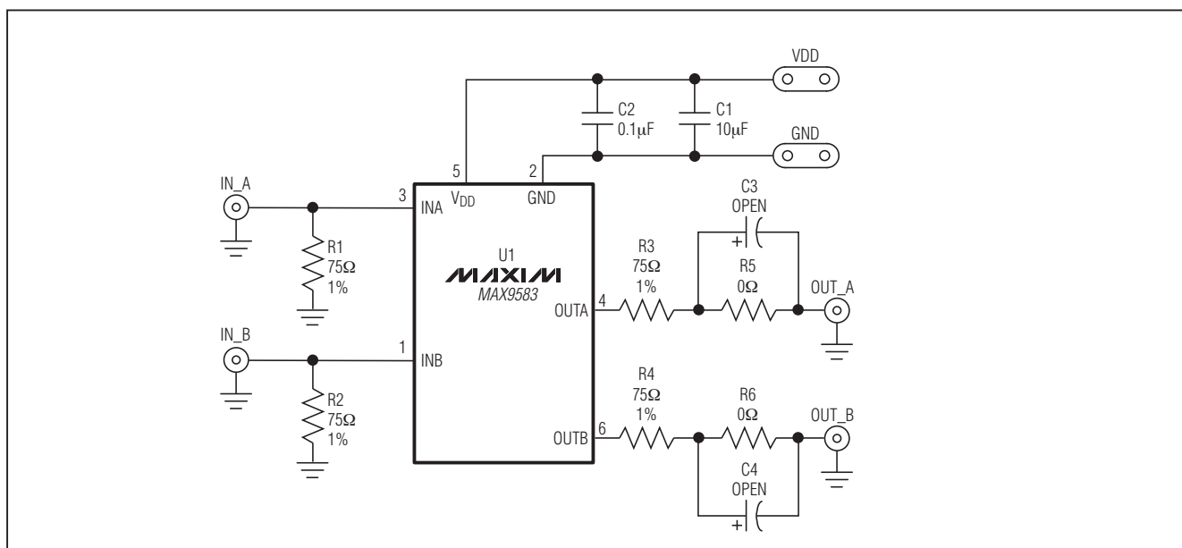
图1. MAX9583评估板原理图
