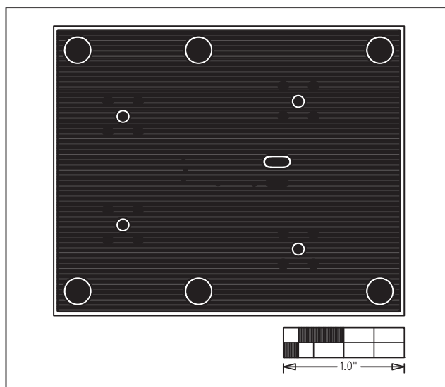
图4. MAX9583评估板PCB布局——焊接层
