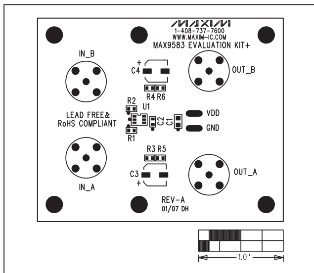
图2. MAX9583评估板元件布局——元件层
