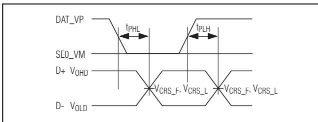
图7. 在DAT_SE0模式下DAT_VP、SEO_VM至D+、D-的时序 (dat_se0 = 1)
