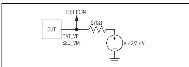
图4. 测量DAT_VP、SEO_VM打开/关闭时间的负载
