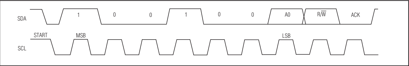
图15. 从设备地址
