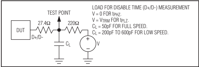
图1. 测量关闭时间的负载
