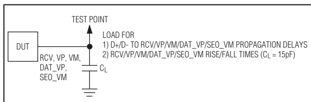
图3. 测量接收机传输延时和接收机上升/下降时间的负载
