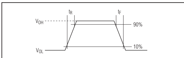
图5. 上升和下降时间
