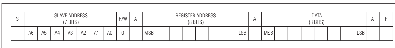
图18. 写字节的格式
