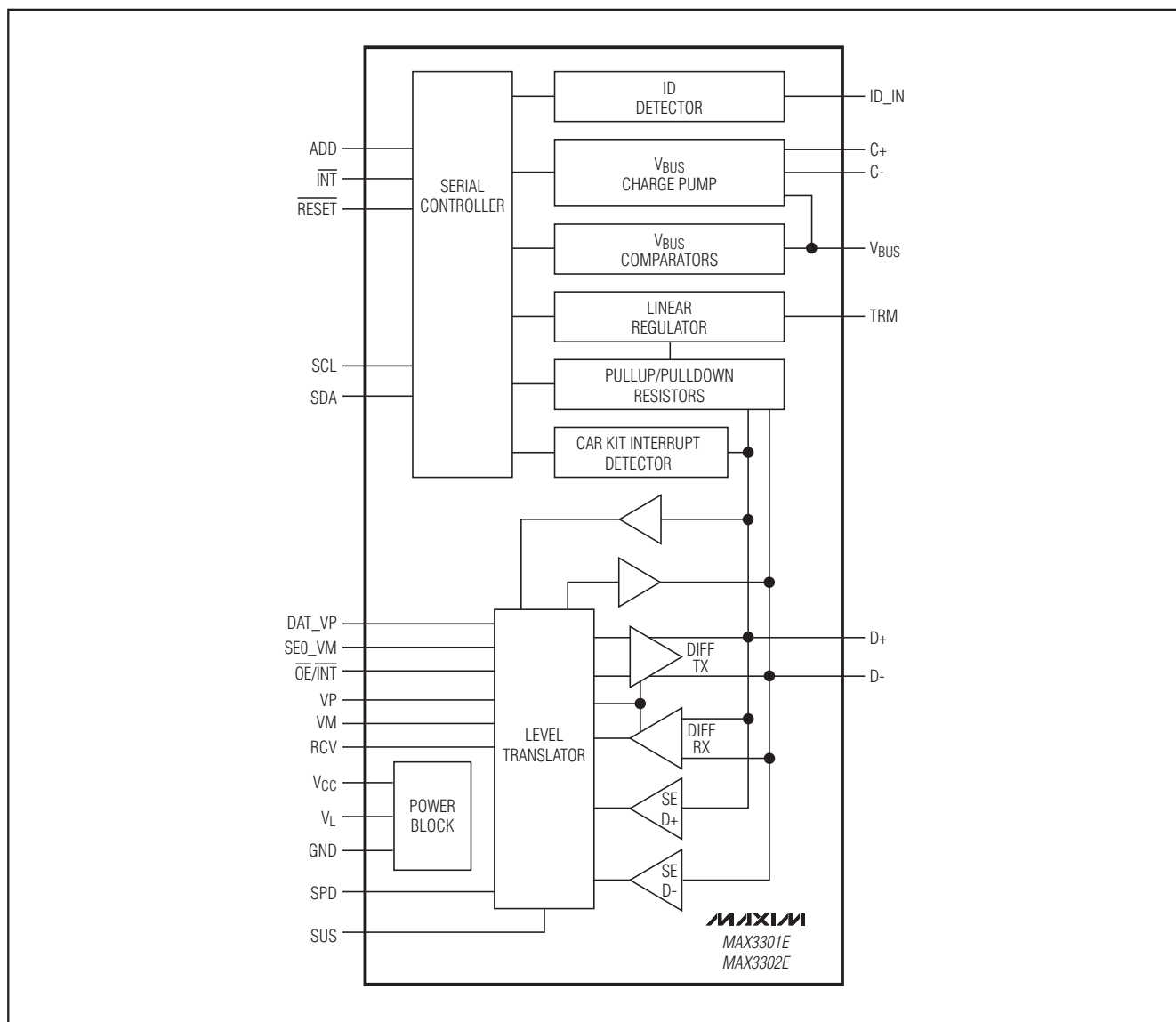
图11. 方框图
