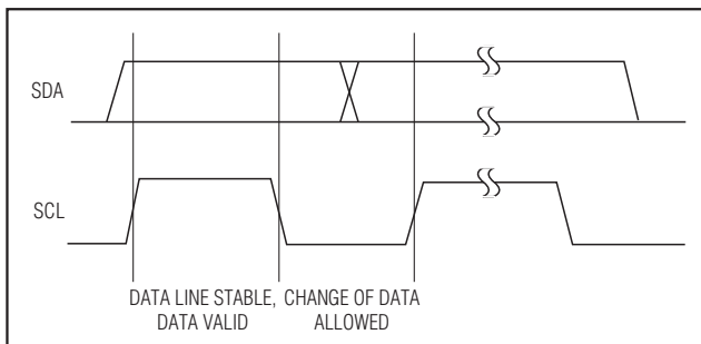
图16. 位传送
