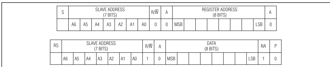
图19. 读字节格式
