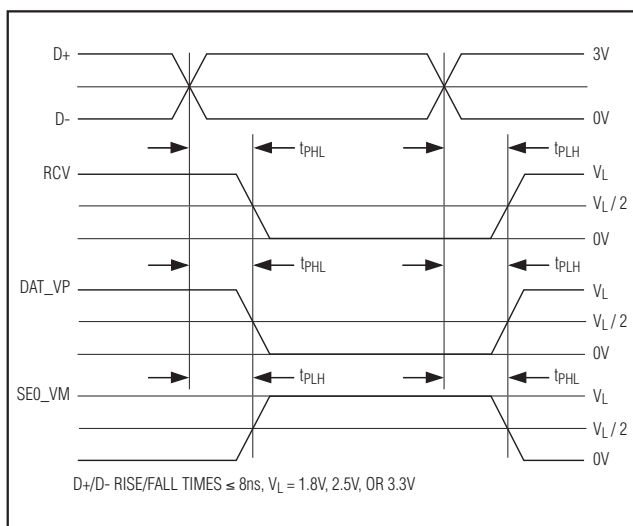
图9. D+/D-至RCV、DAT_VP、SEO_VM传输延时(VP_VM模式)
