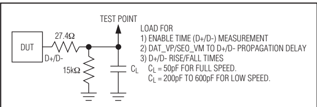
图2. 测量打开时间、发送器传输延时和发送器上升/下降时间的负载
