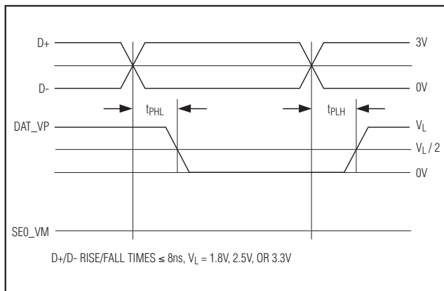
图10. D+/D-至DAT_VP、SEO_VM传输延时(DAT_SE0模式)
