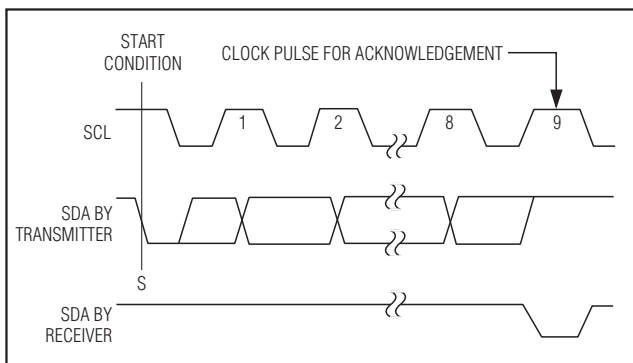
图17. 应答
