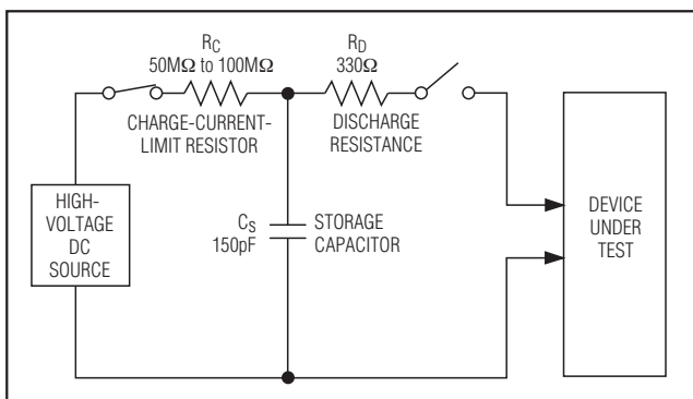
图24. IEC 61000-4-2 ESD测试模型
