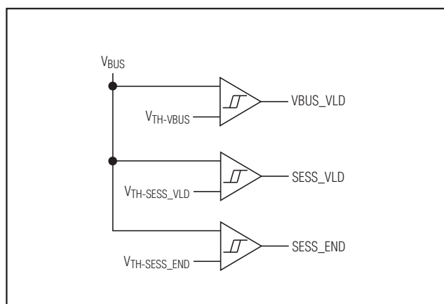
图12. 比较器网络框图
