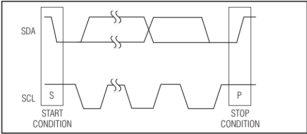
图14. 开始和停止状态
