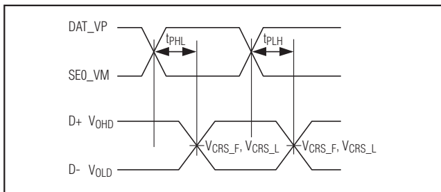
图6. 在VP_VM模式下DAT_VP、SEO_VM至D+、D-的时序 (dat_se0 = 0)
