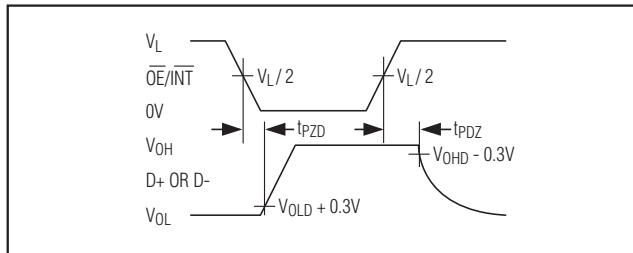
图8. 打开和关闭时序
