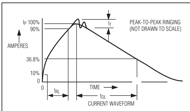
图23. 人体模型电流波形
