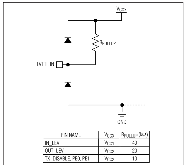
图7. LVTTTL等效输入结构
