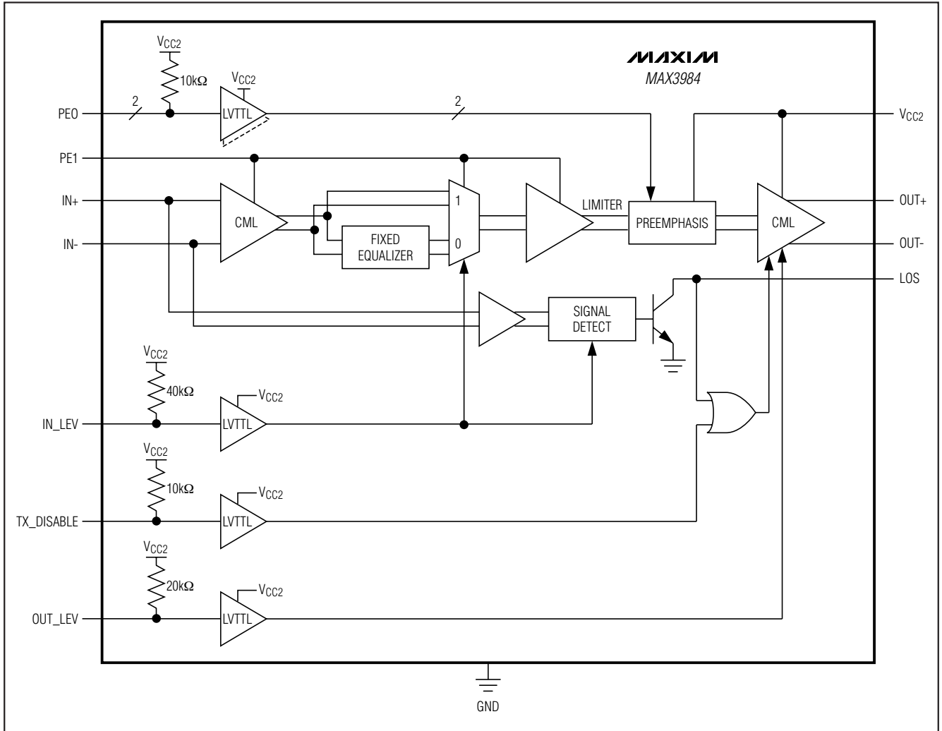
图4. 功能框图
