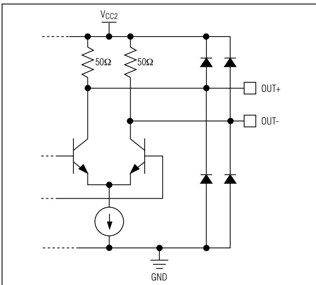
图6. OUT+/OUT-等效输出结构
