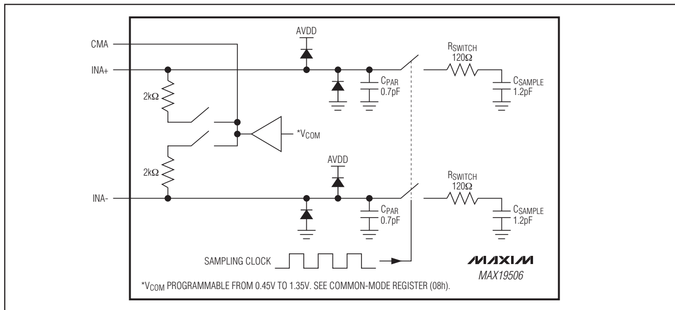
图3. 内部采样保持(T/H)电路
