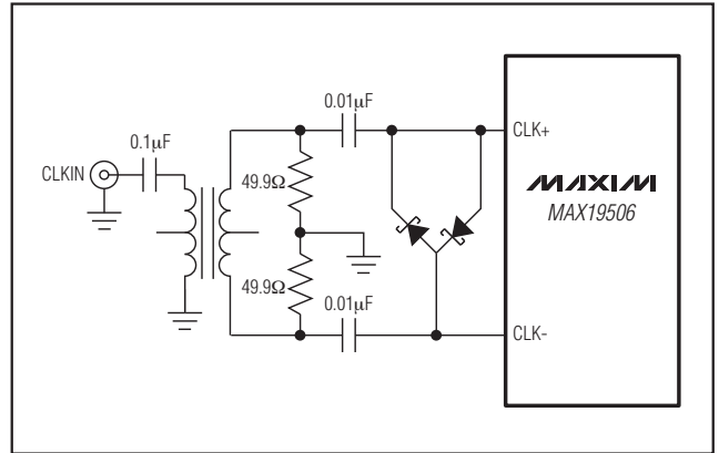
图21. 单端至差分时钟输入
