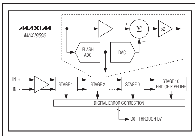
图1. 流水线结构——分级框图
