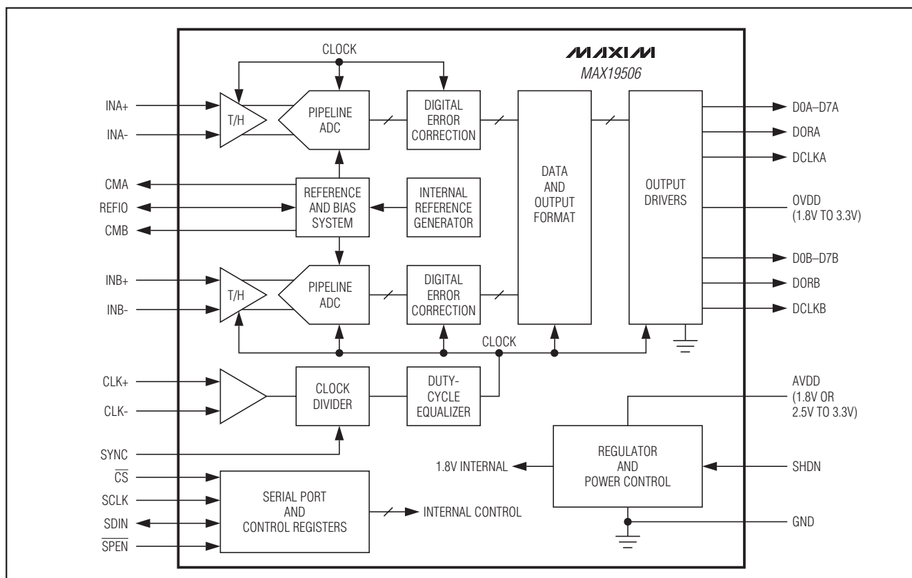
图2. 功能框图
