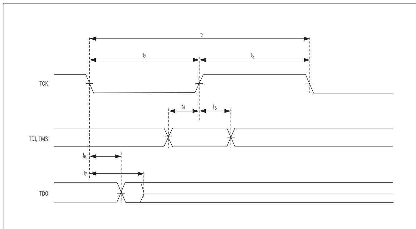
图2. JTAG时序图
