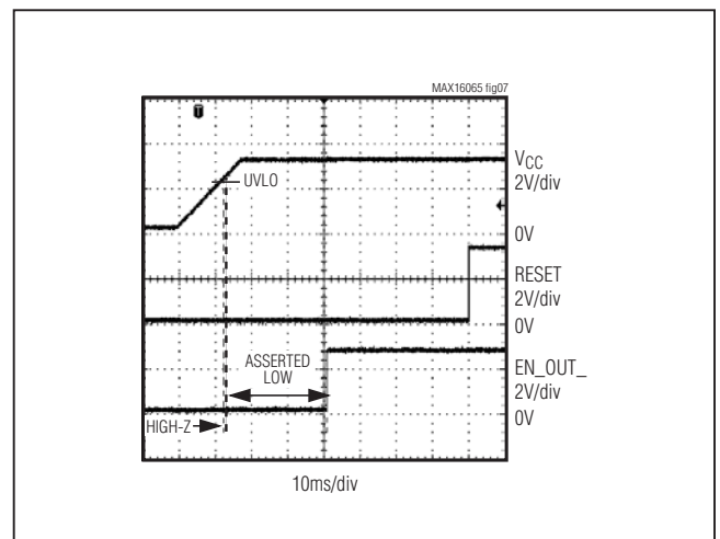
图7. 上电过程中的RESET和EN_OUT_，EN_OUT_ 配置为推挽式高电平有效输出
