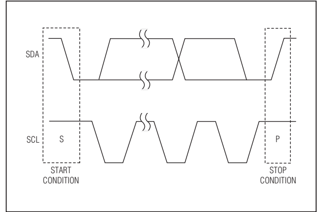
图12. START和STOP条件
