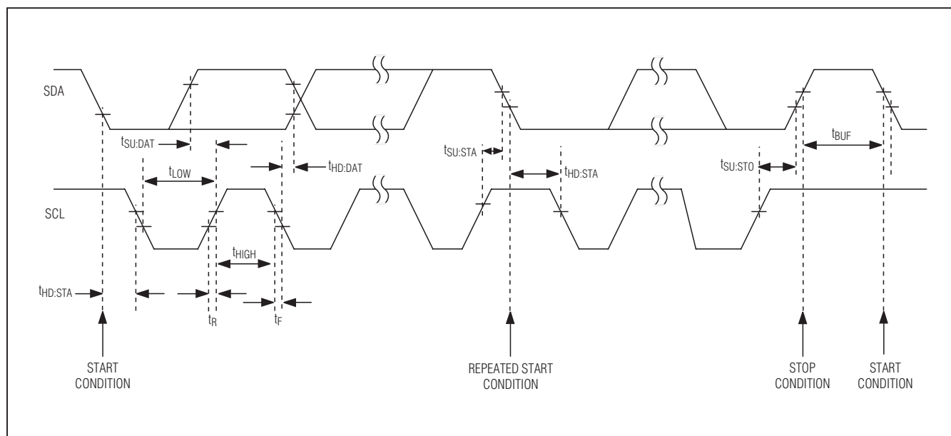
图1. SMBus时序图
