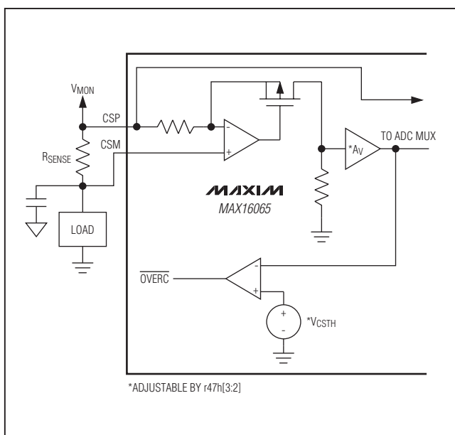
图5. 检流放大器
