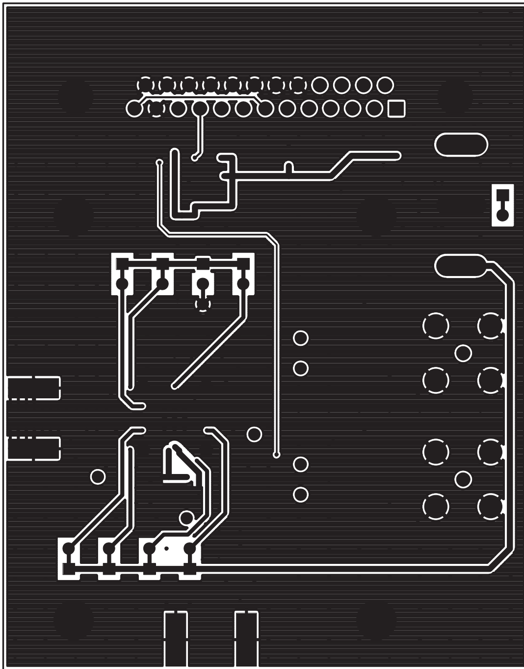
图4. MAX2120评估板PCB布局—底层
