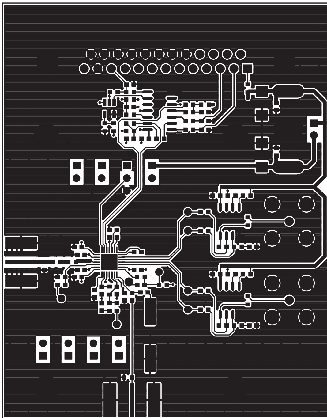
图3. MAX2120评估板PCB布局——顶层
