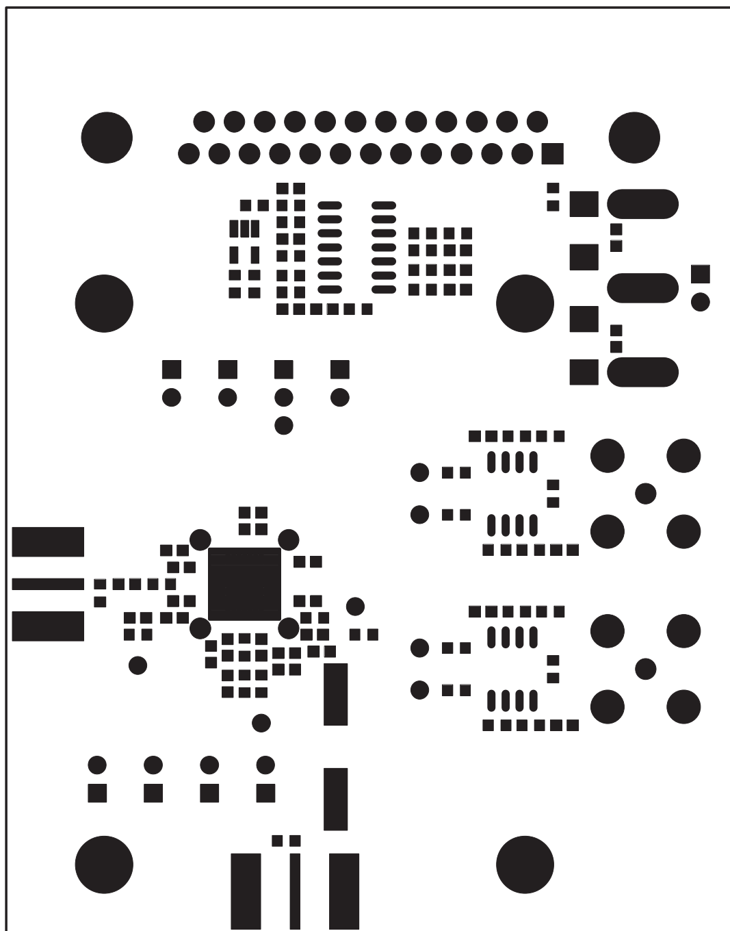
图5. MAX2120评估板PCB布局—顶层阻焊层
