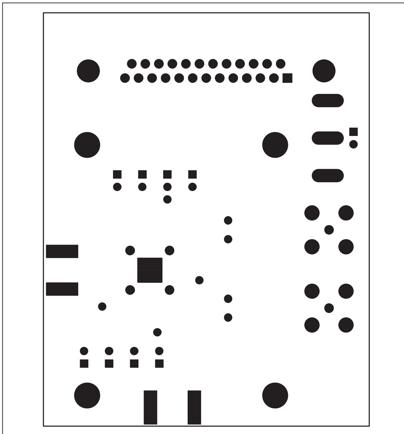
图6. MAX2120评估板PCB布局—底层阻焊层
