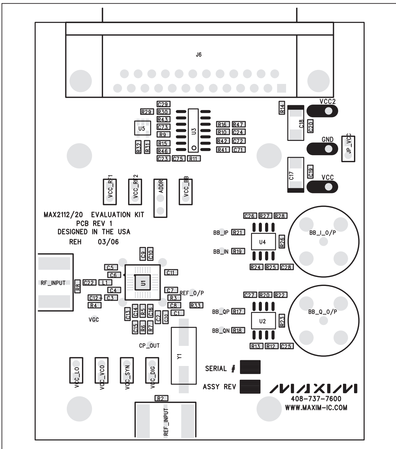
图2. MAX2120评估板PCB布局——元件布局
