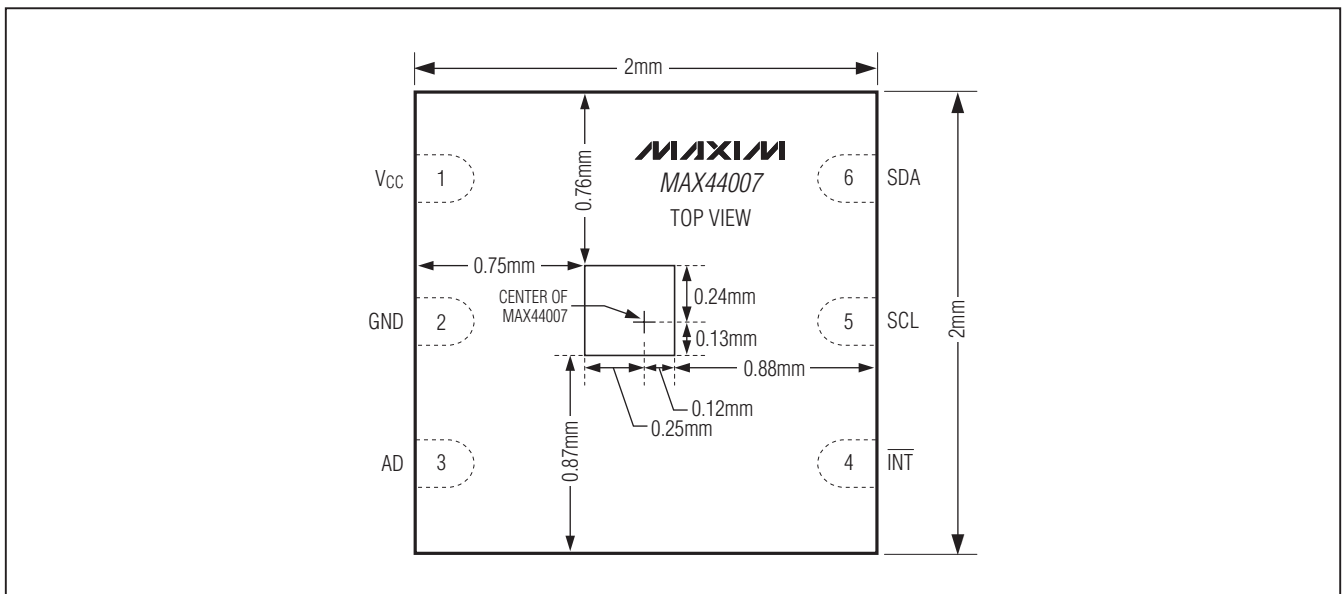
图8. 传感器位置
