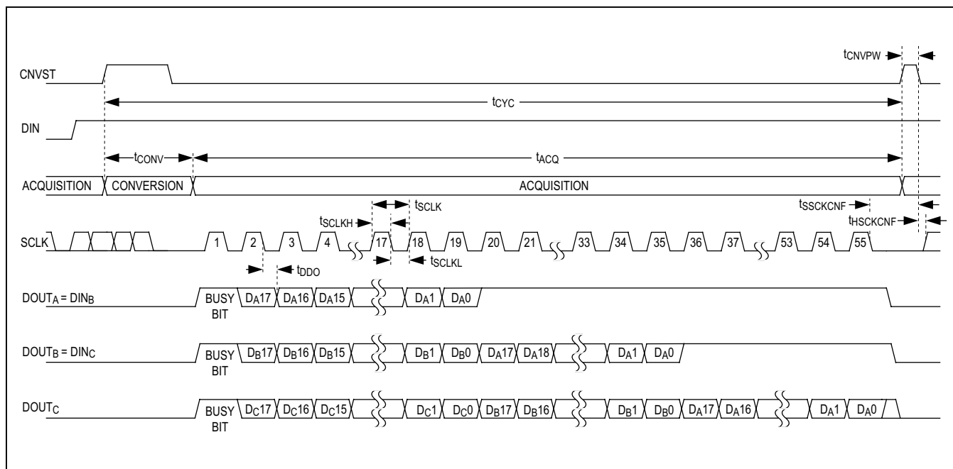
图15. 带“忙”指示菊链模式时序图
