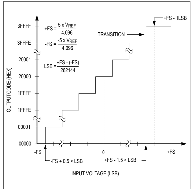
图3. 双极性传递函数
