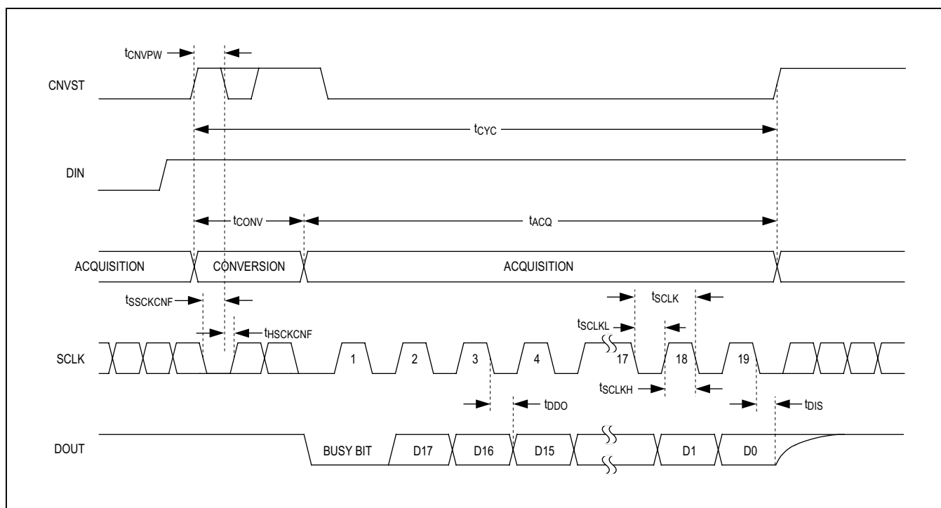
图9. 带“忙”指示CS模式工作时序
