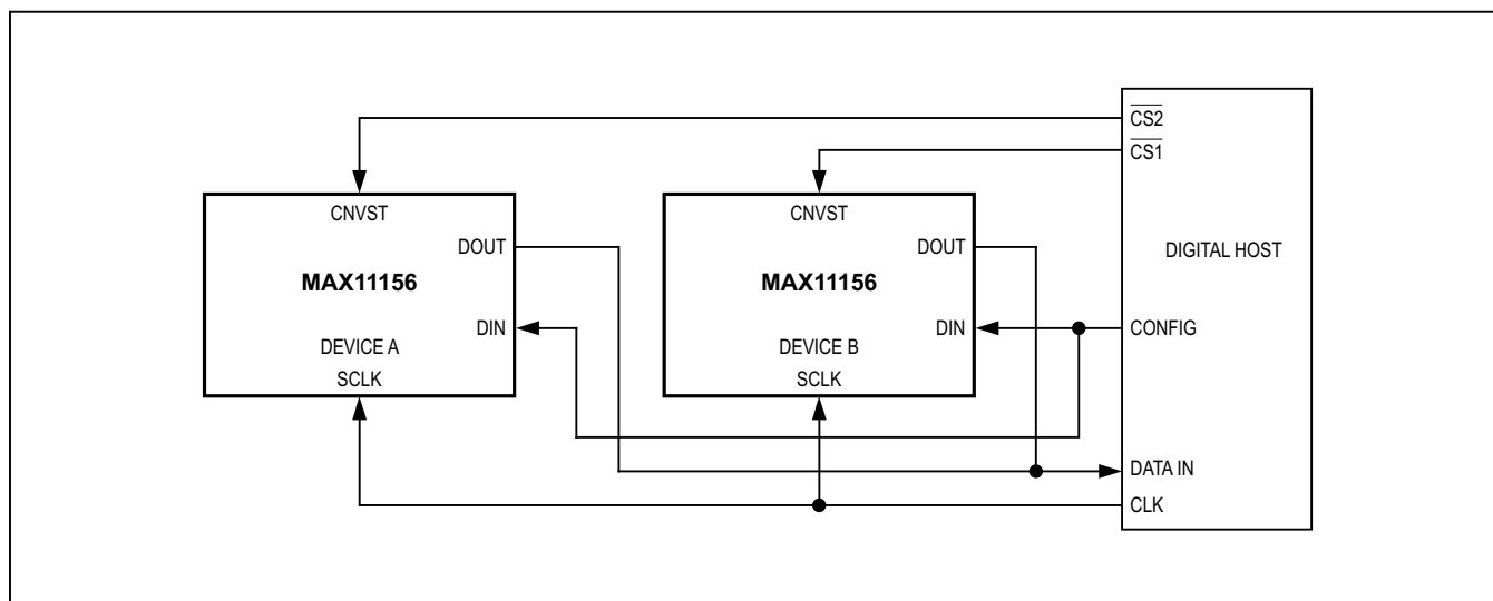
图10. 多通道 \overline{CS} 配置图
