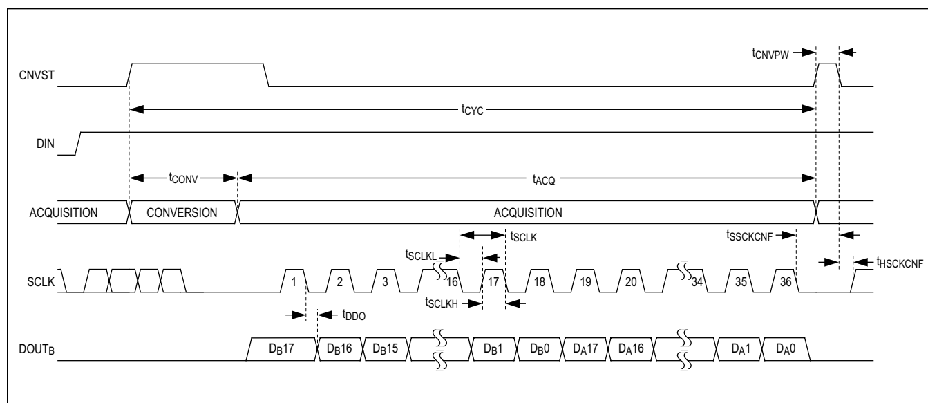
图13. 无“忙”指示菊链模式时序图
