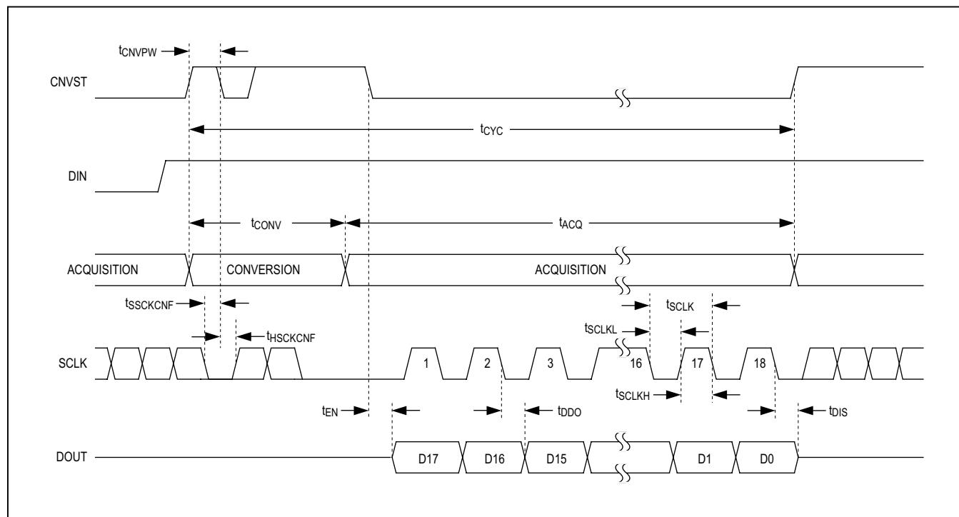
图7. 无“忙”指示 \overline{CS} 模式工作时序
