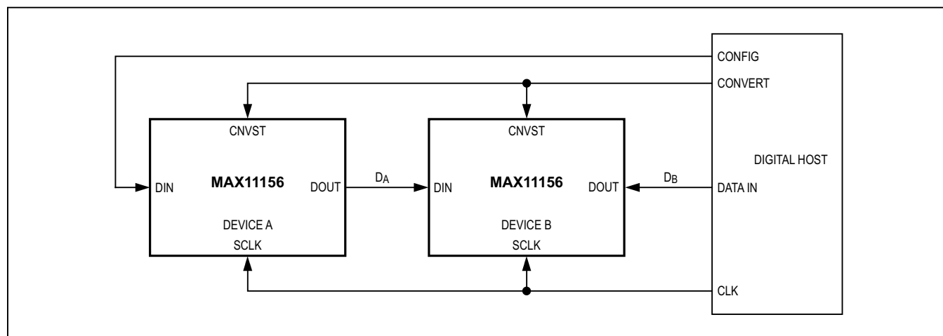
图12. 无“忙”指示菊链模式连接图
