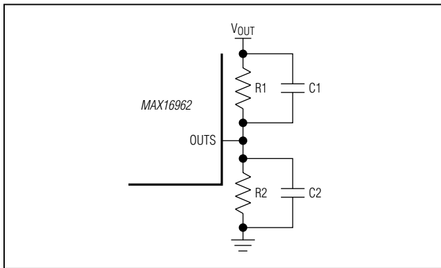
图2. 可调输出电压设置
