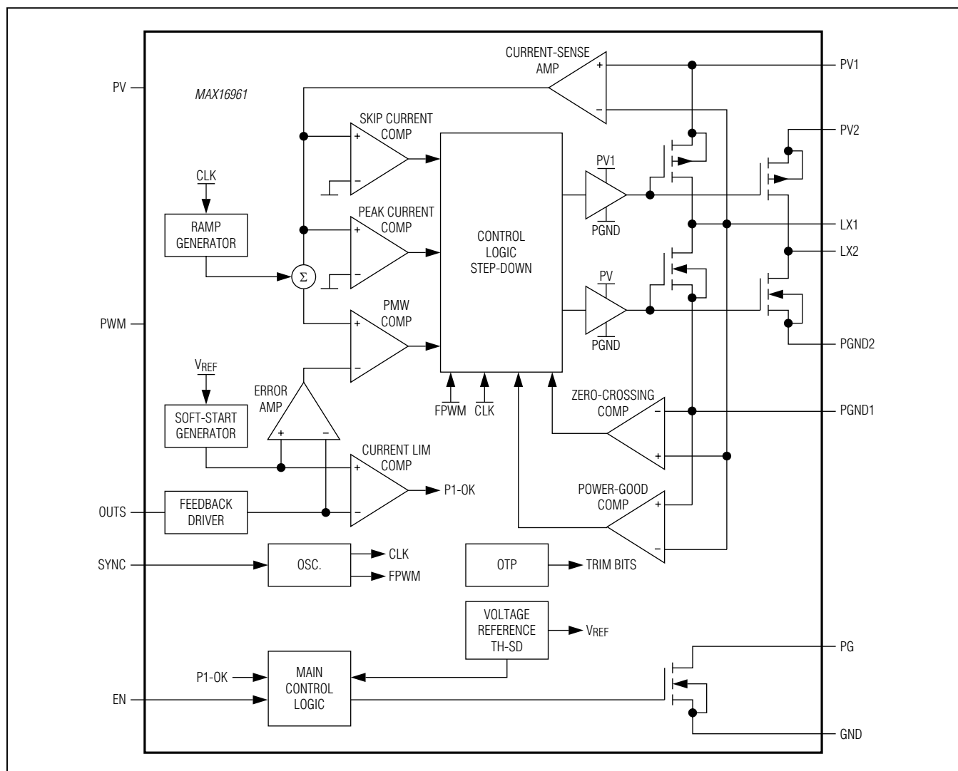
图1. 内部框图
