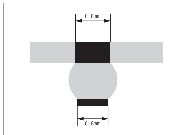
图3. WLP焊球尺寸
