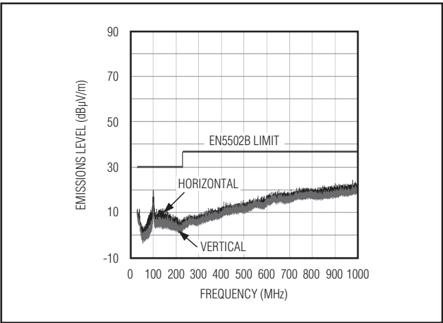
图1. 采用60cm扬声器电缆、无输出滤波器时的EMI特性
