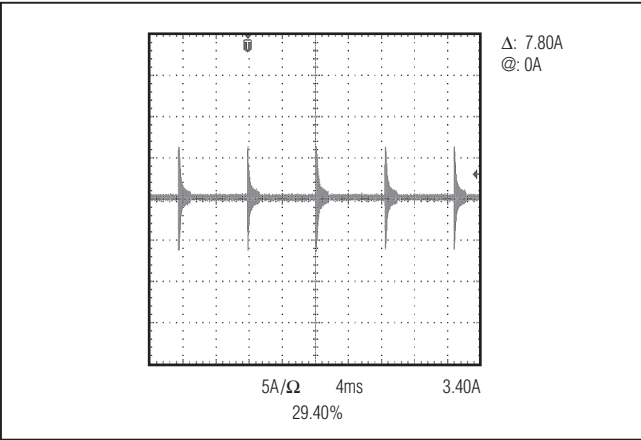
图1. 采用电子变压器(Lichtech LET60)条件下的LED电流波形
