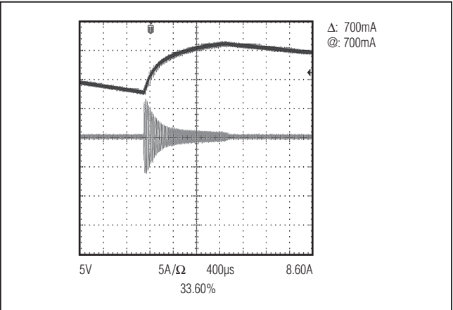
图3. 配合电子变压器(Lichtech LET60)工作时的性能 (CH1: 输入电解电容C1两端的电压波形; CH4: 输入电流波形)
