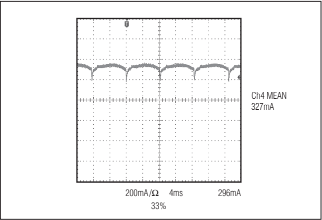
图2. 采用电子变压器(Lichtech LET60)条件下的输入电流波形
