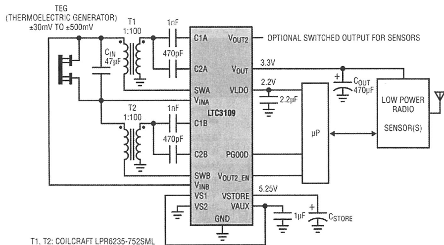
图 2：针对单极输出操作的 LTC3109 原理图
